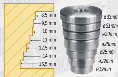
Schéma 7 : largeur d'usinage obtenue avec chacun des roulements.
