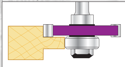
Schéma 17 : usinage d'une languette (ou d'un tenon) centré.
