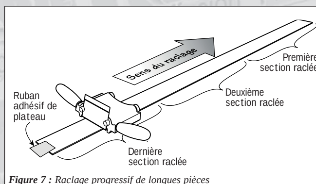
Figure 7 : Raclage progressif de longues pièces
