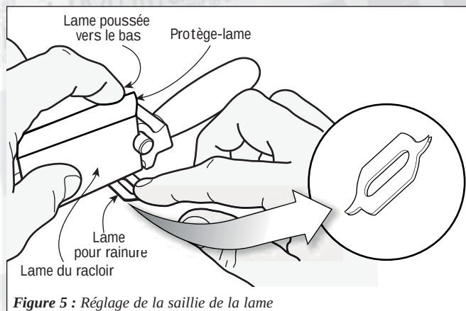
Figure 5 : Réglage de la saillie de la lame
